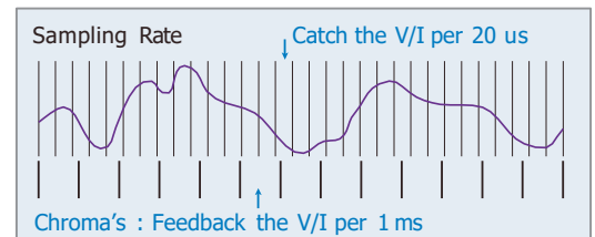
クロマ充電試験システムのサンプリングレート
