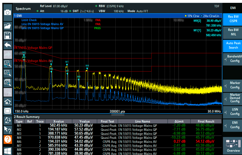
R&S®FPL1-K54 EMI測定アプリケーション
