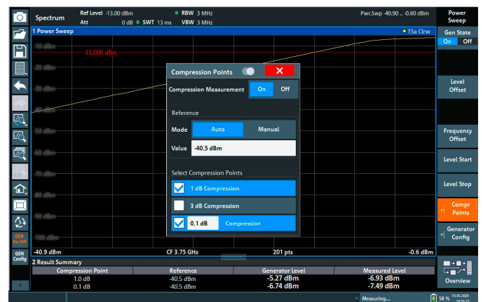
1 dBおよび0.1 dB圧縮ポイントの測定
