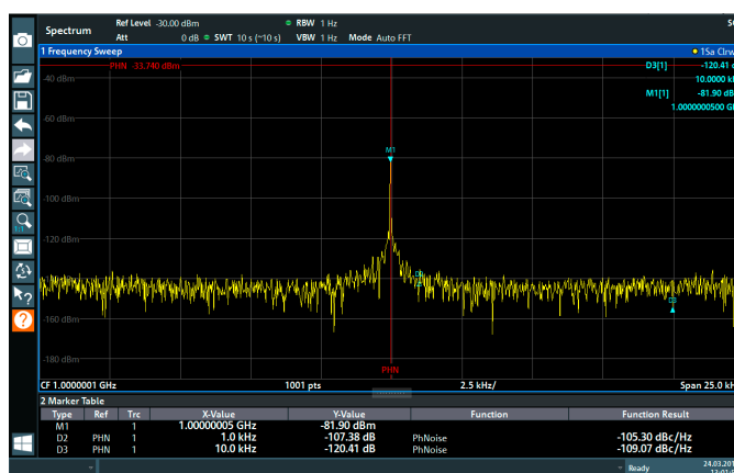
マーカー機能によるシンプルな位相雑音測定
